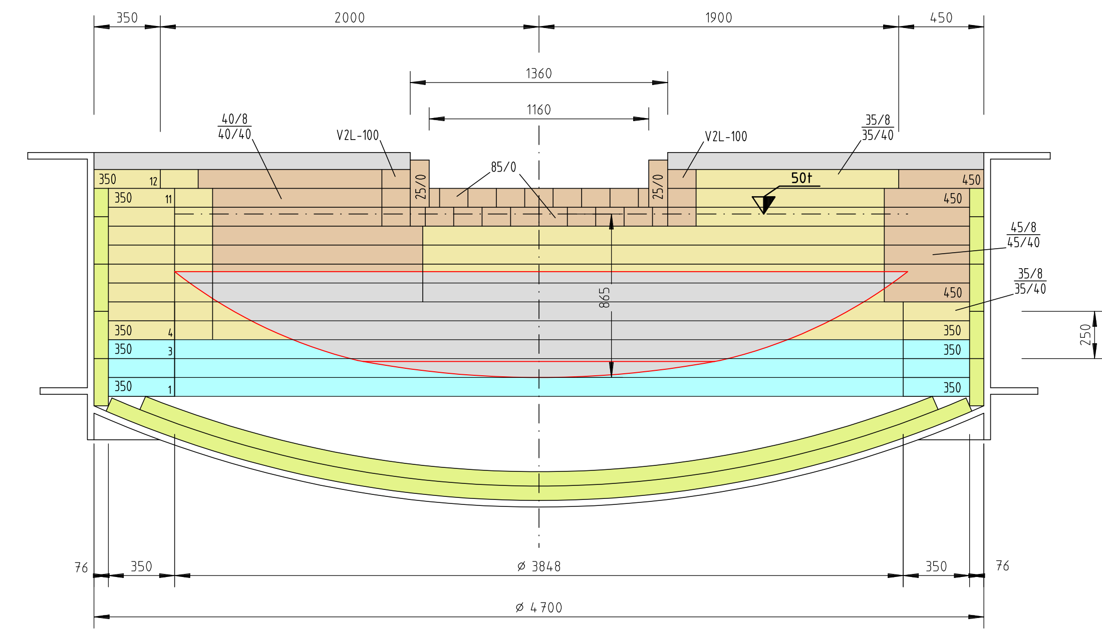
Schnitt D-D
