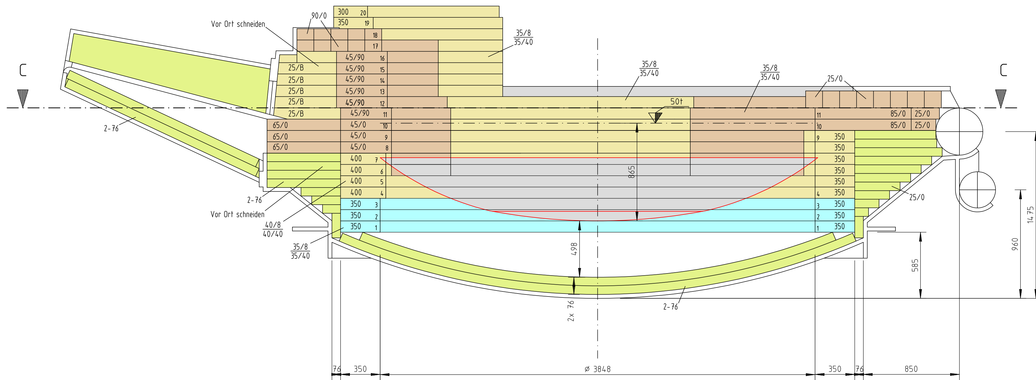
Schnitt A-A
