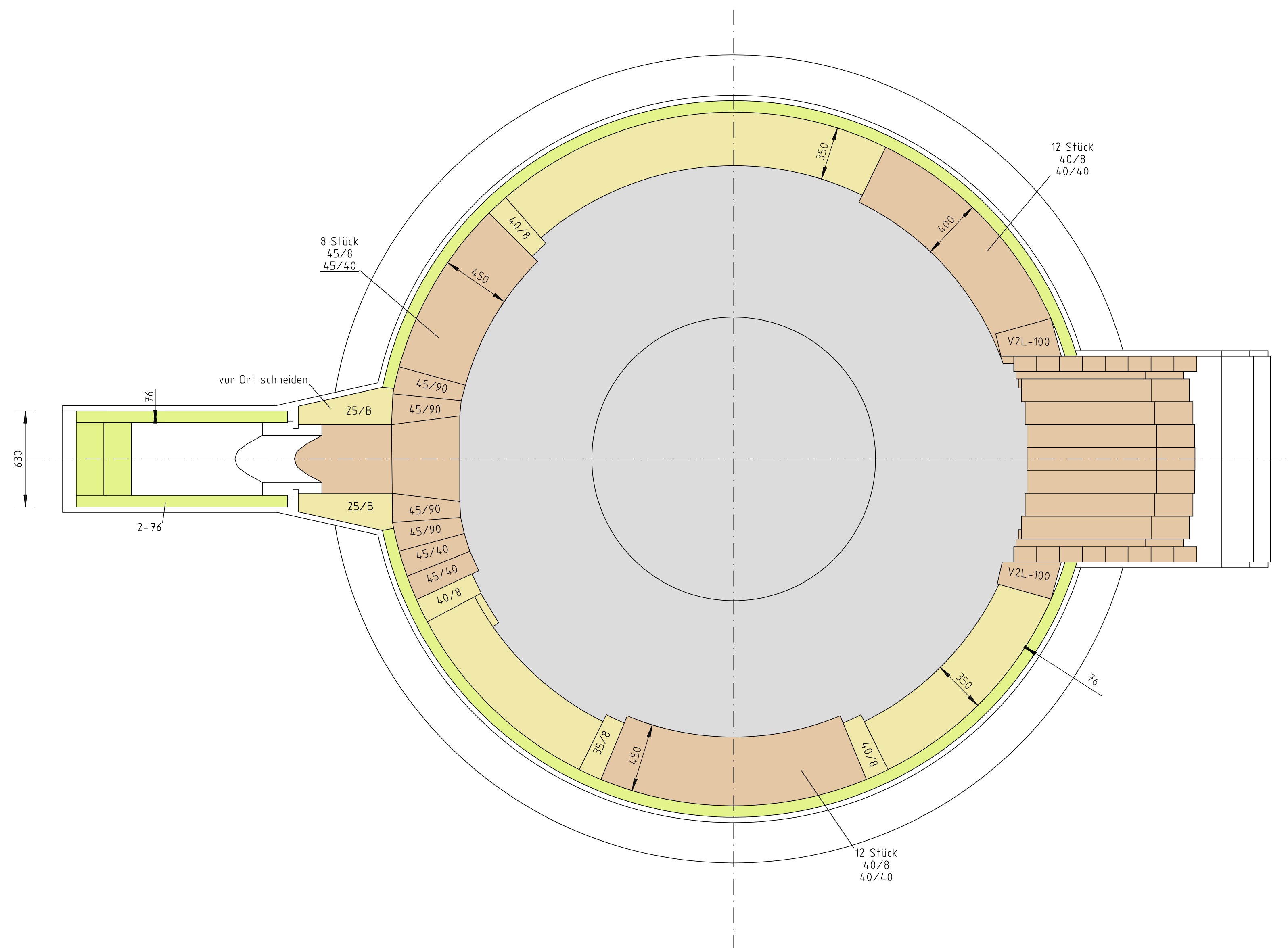
Schnitt C-C Lage 11
